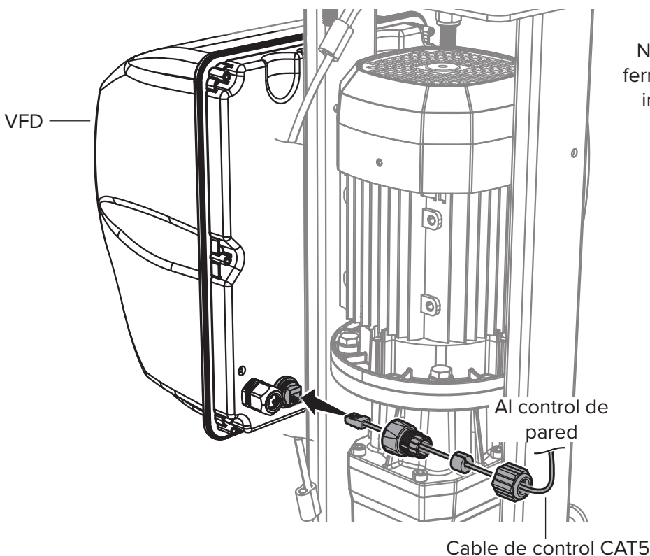
Fig. 1: Cable de control CAT5 al VFD
