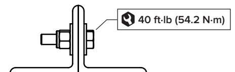
Vista lateral
