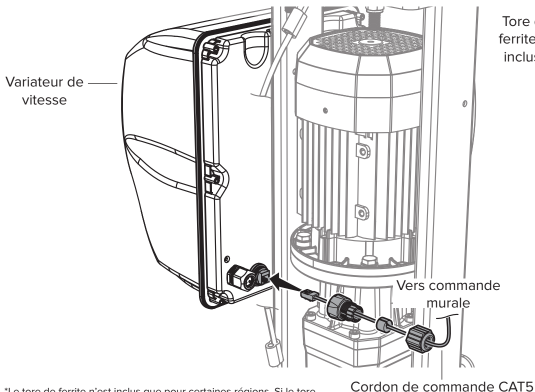
Fig. 1 : Cordon de commande CAT5 vers variateur de vitesse
