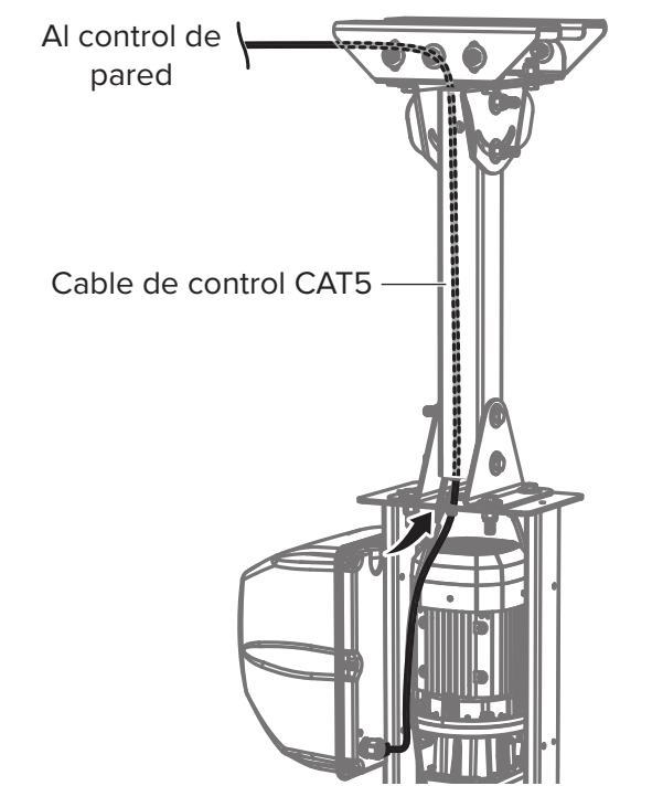
Fig. 2: Tendido del cable de control CAT5
