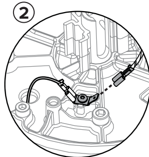
Connect Earth/ Ground Wire Connectez le fil de terre Conectar el cable de tierra
