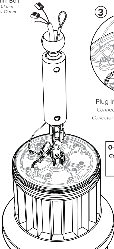
Connect Safety Cable Raccordez l'élingue de sécurité Conectar el cable de seguridad
