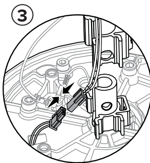
Plug In Wiring Harnesses Connectez les faisceaux de fils Conectar los arneses del cableado
